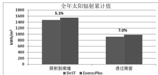
图 11 照射到南墙和透过窗户的全年太阳辐射累计值
