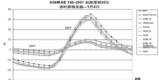
图6 算例600FF和900FF逐时基础室温
