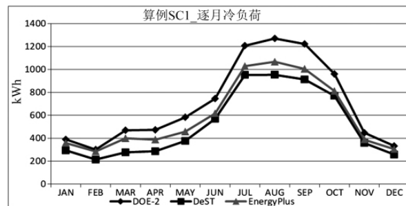
图 21 算例 SC1 逐月冷负荷
