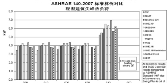
图5 算例600-650全年尖峰热负荷
