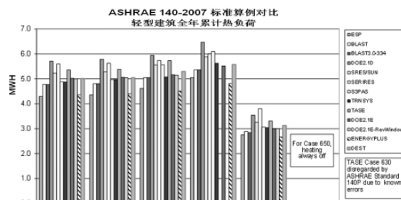
图4 算例600-650全年累计热负荷
