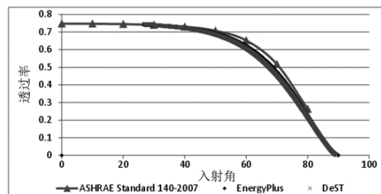
图 12 不同入射角下的太阳辐射透过率
