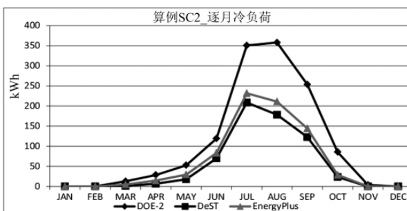
图 22 算例 SC2 逐月冷负荷
